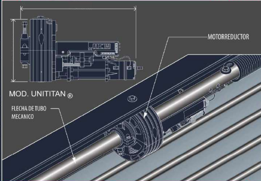
3 MOTOR ELECTRICO INTERNO
