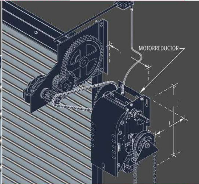
4 MOTOR ELECTRICO EXTERNO
