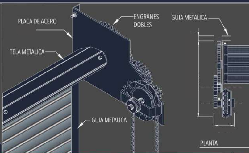
2 APARATO DE CADENA
